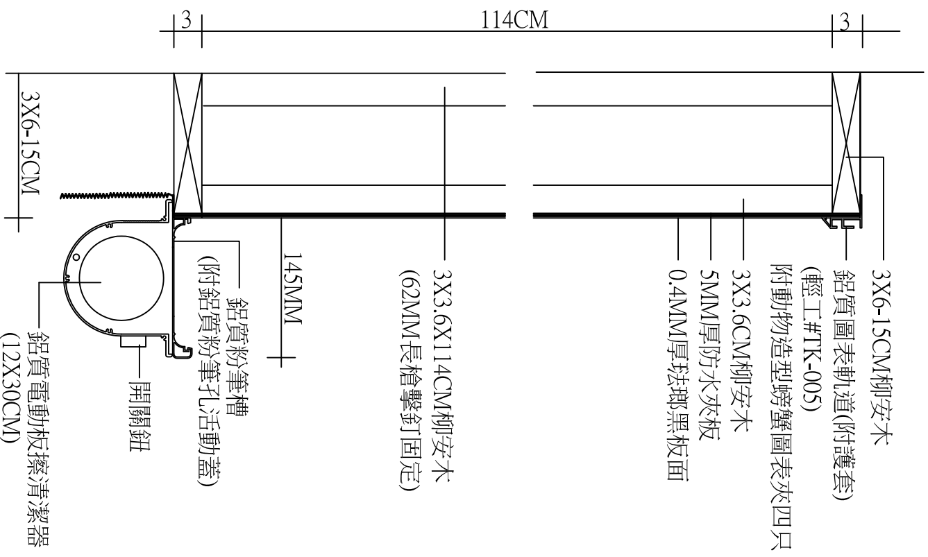
立面圖 S:1/5
