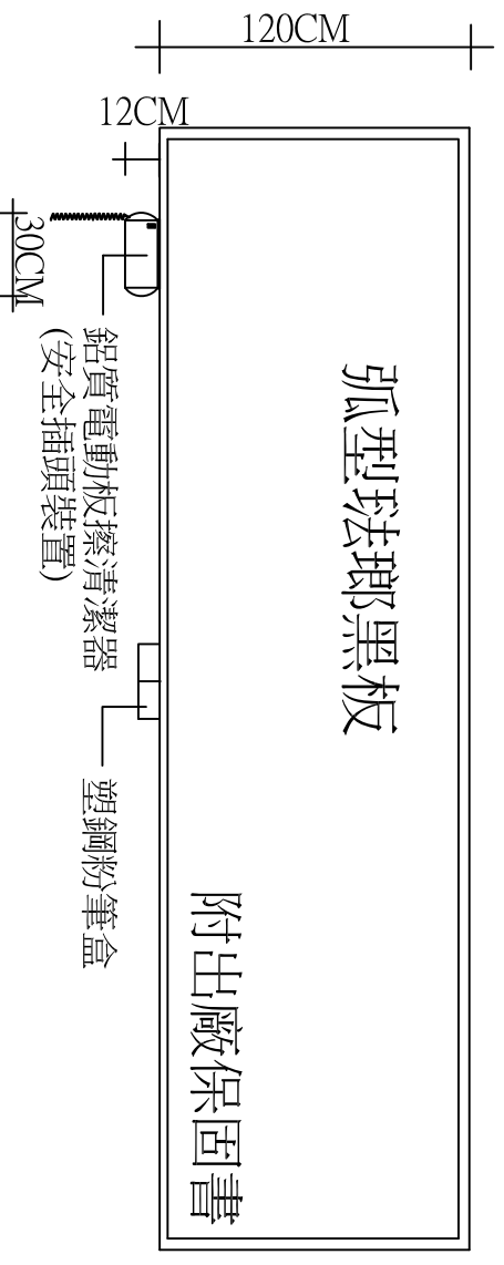
正面圖 S:1/30
