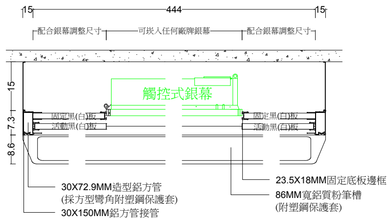
平面圖 S : 1/5
