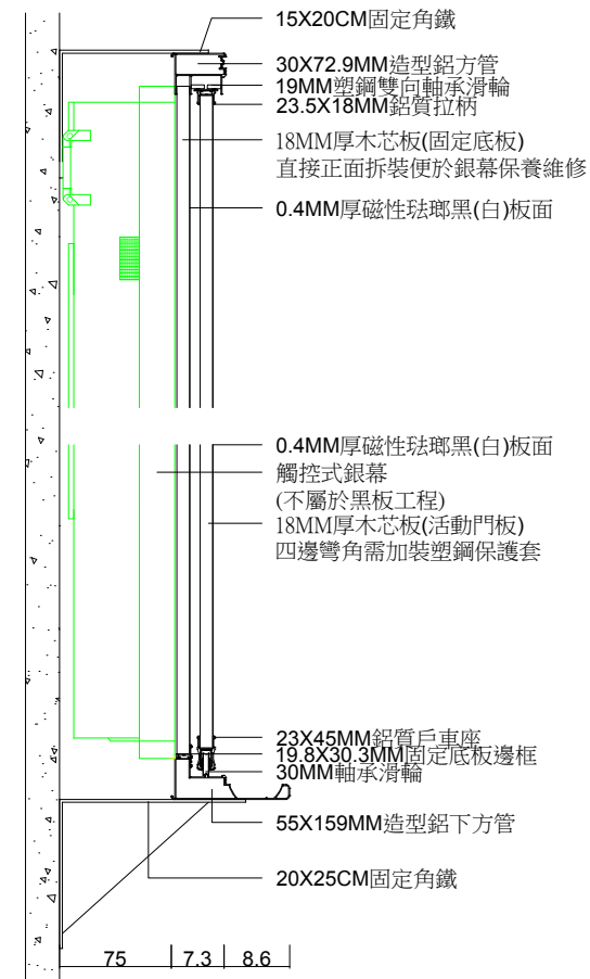
立面圖 S : 1/5
