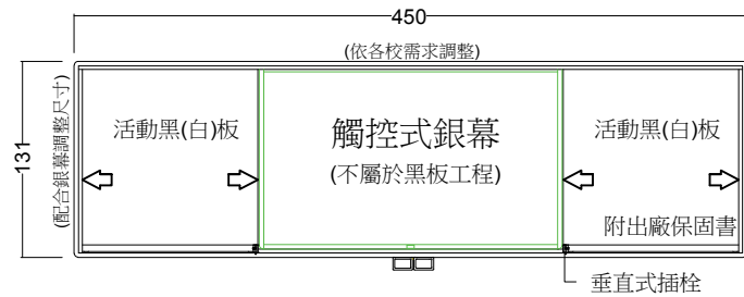
正面圖
