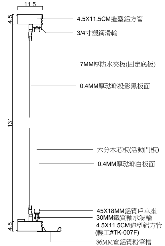
立面圖 S:1/5
