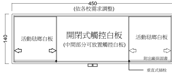
正面圖
