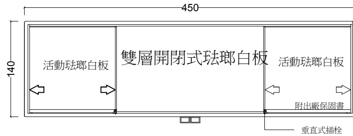
正面圖
