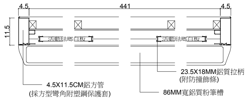
平面圖 S:1/5
