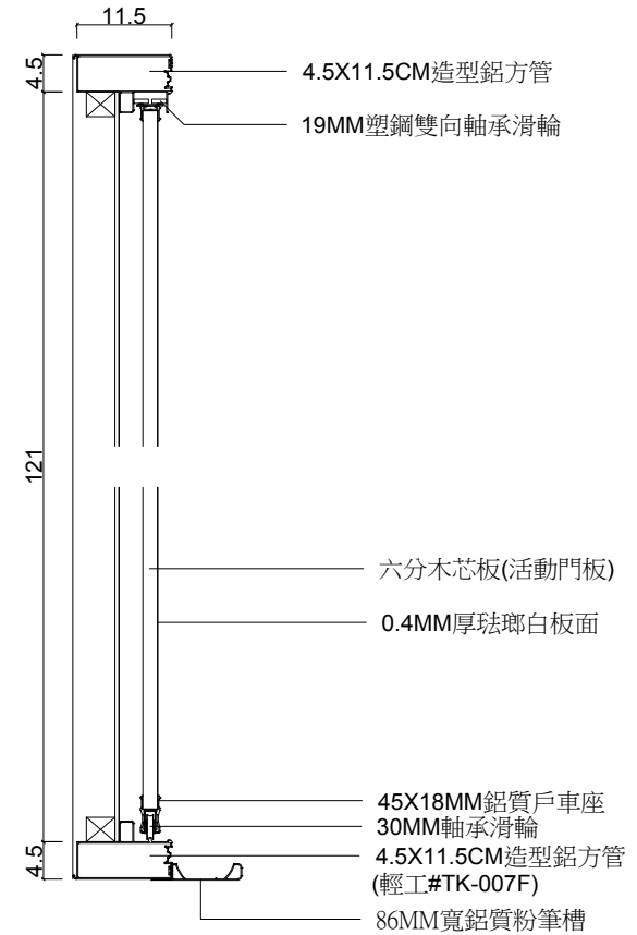
立面圖 S:1/5
