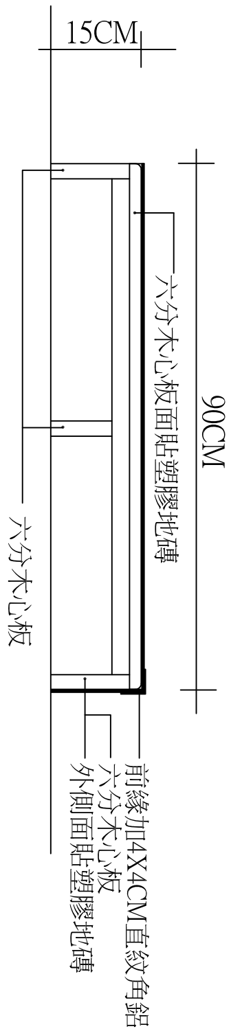
平面圖 S:1/5
